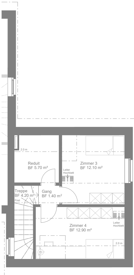
Dachgeschoss
